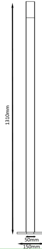
zappi Abmessungen
