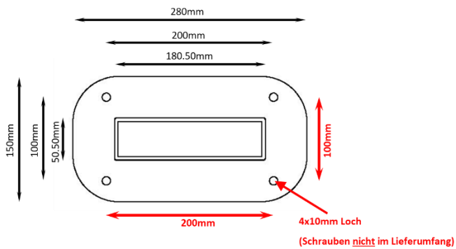
Grundplatte
